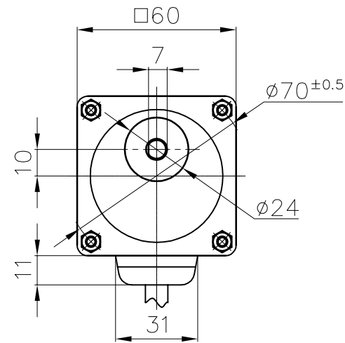
A矢視図
